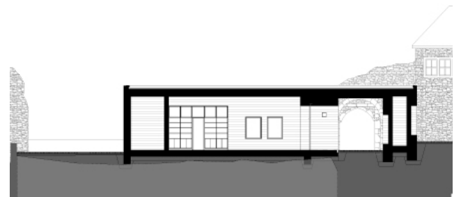
Schnitt
