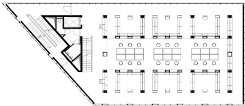
Grundriss Obergeschoss
