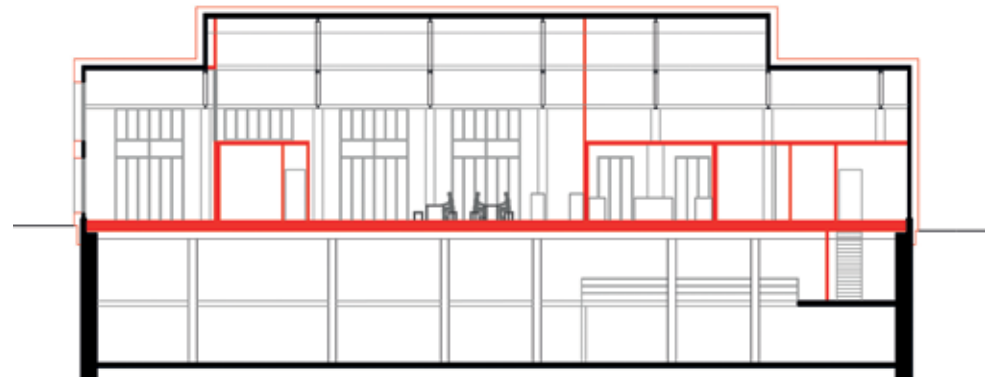
Schnitt
