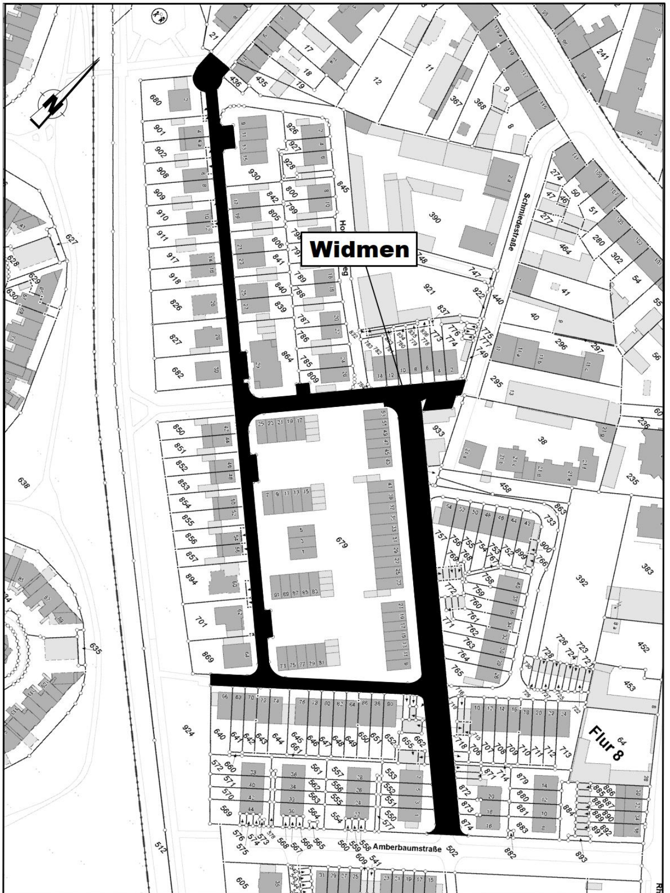
Referat Vermessung und Kataster, Fiederblattweg, Gelsenkirchen
