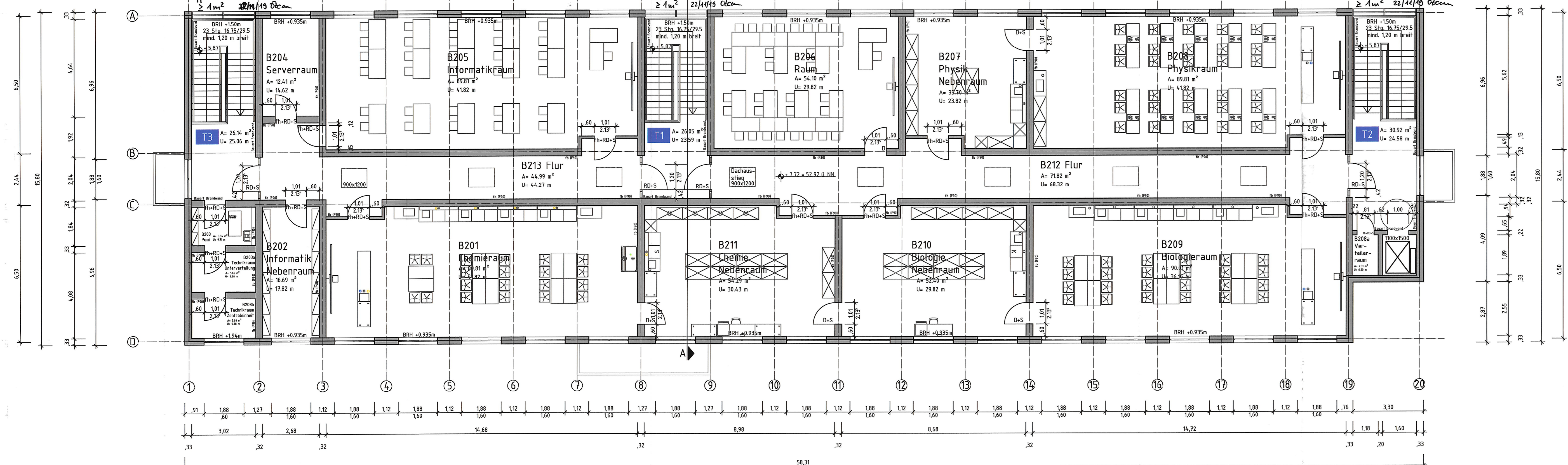
Grundrisse EG - 2.OG M 1:100
